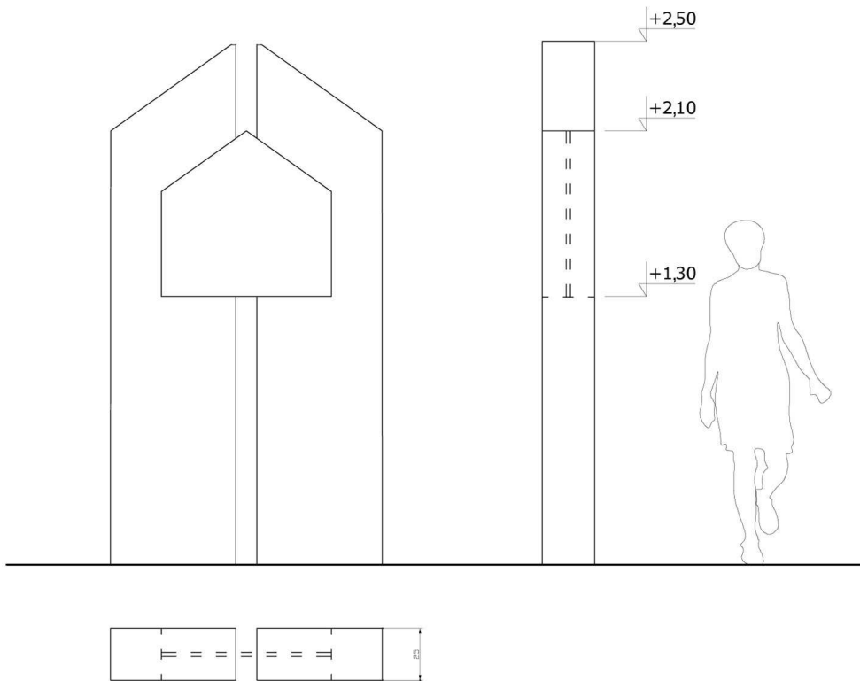
Kapliczka – schemat - elewacja frontowa.
